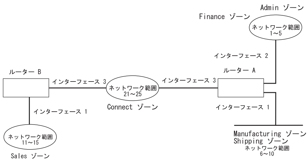
図 12. ゾーン・フィルター処理の例
