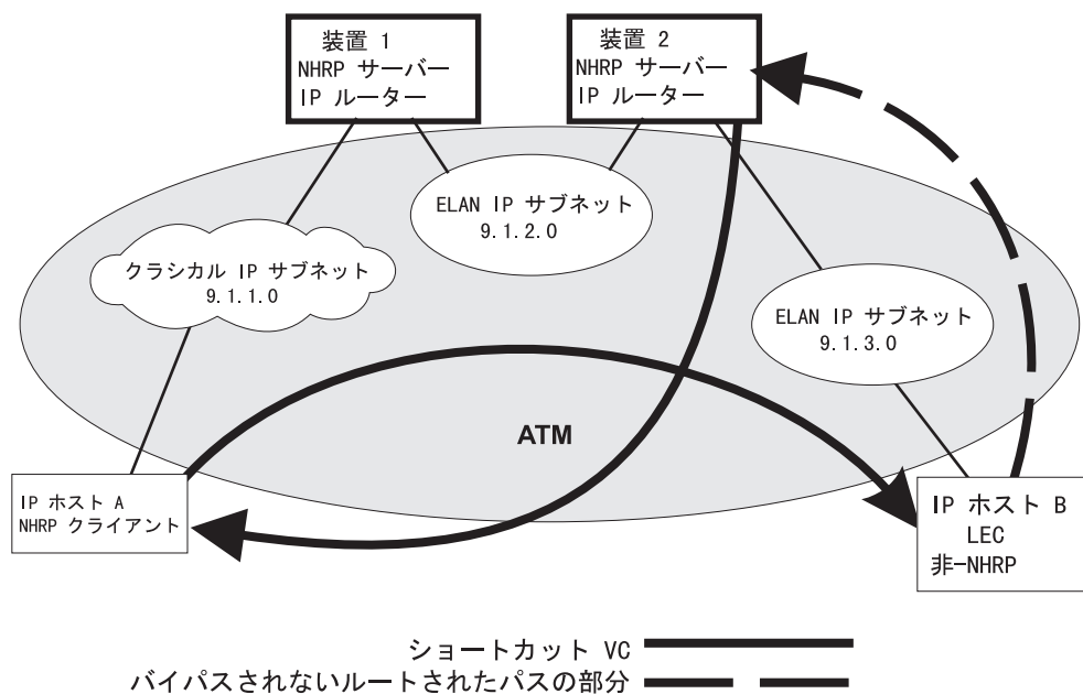
図 32. 混合されたクラシカル IP および ELAN 環境における NHRP
