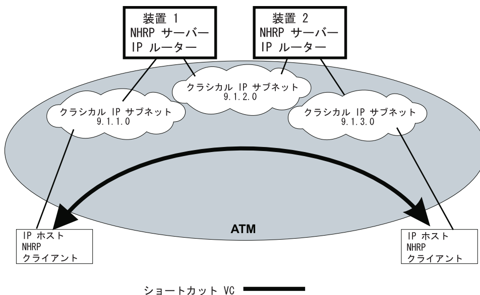
図 28. クラシカル IP 環境における NHRP
