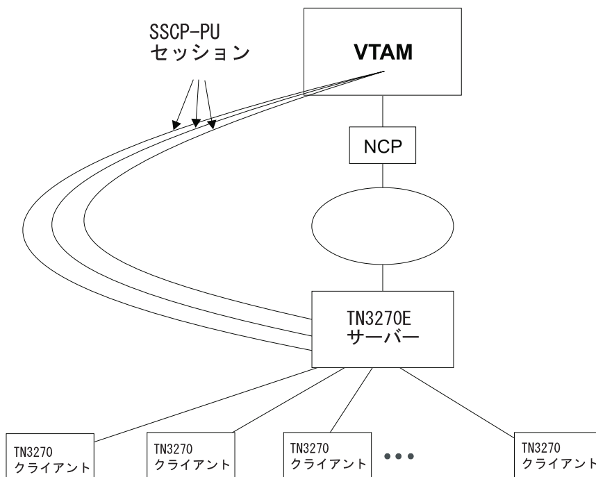
図2. サブエリアに接続された SNA ノード用の複数の PU
