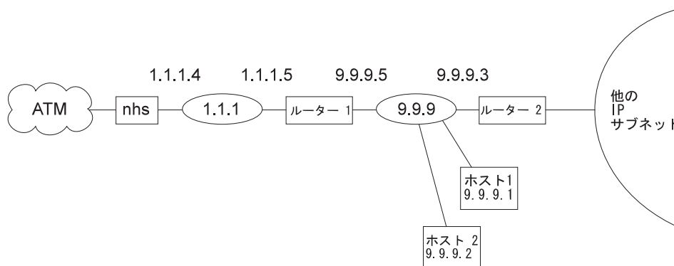
図 34. 不許可ルーター間ショートカットの使用
