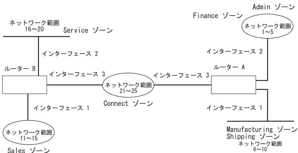
図13. ネットワーク・フィルター処理の例
