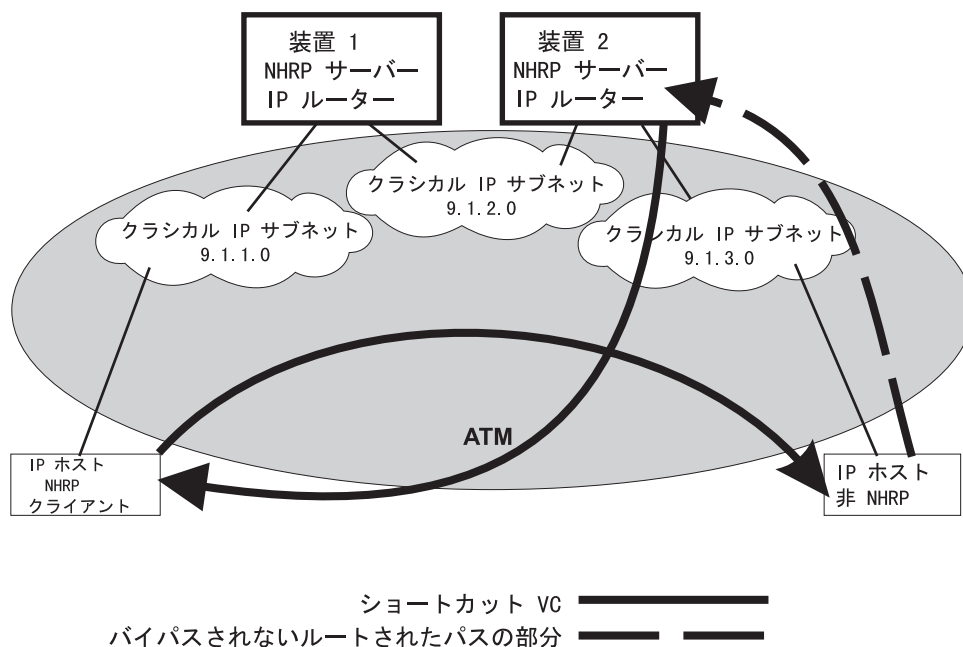
図 29. 非 NHRP 装置をもつクラシカル IP 環境における NHRP
